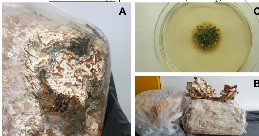
Immagine 1. A. Balla con sintomi da muffa verde. B. Balle analizzate. C. Isolato da Trichoderma sp.
