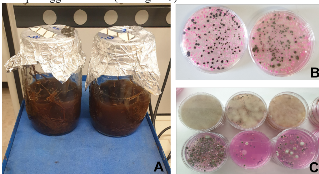
Immagine 3. Metodo de isolamento A. Campioni di composto in agitazione. B e C. Diluzioni seriali in terreno semiselettivo.
