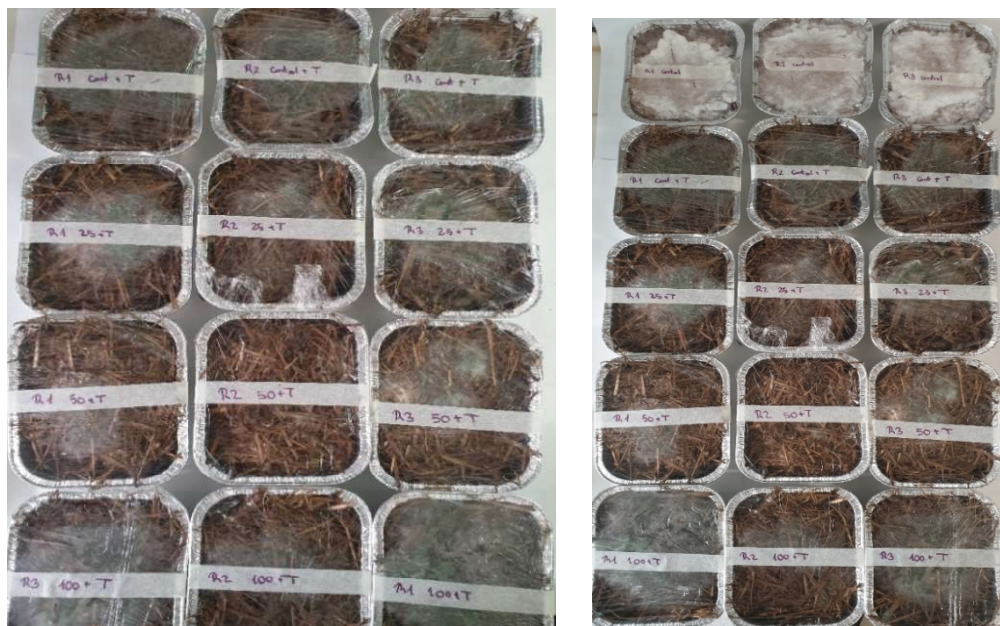
Immagine 6. Vaschette dopo 10 giorni di incubazione a 28°C inoculate con micelio di Pleurotus e Trichoderma
